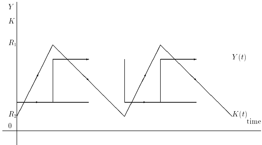
図 8.4: グッドウィンのモデル 1 の動き
