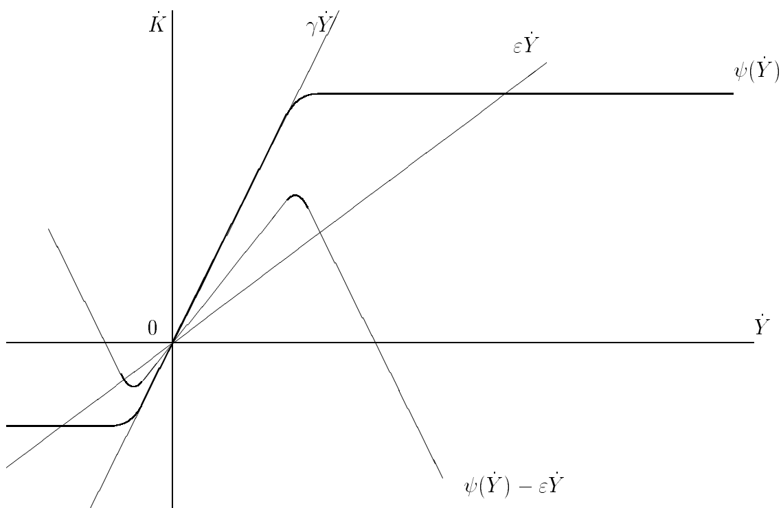
図 8.5: グッドウィンの非線形加速度因子
