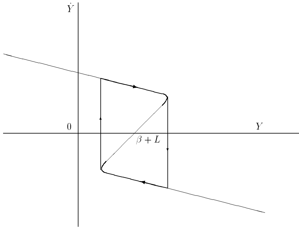
図 8.6: グッドウィンのモデルの位相
