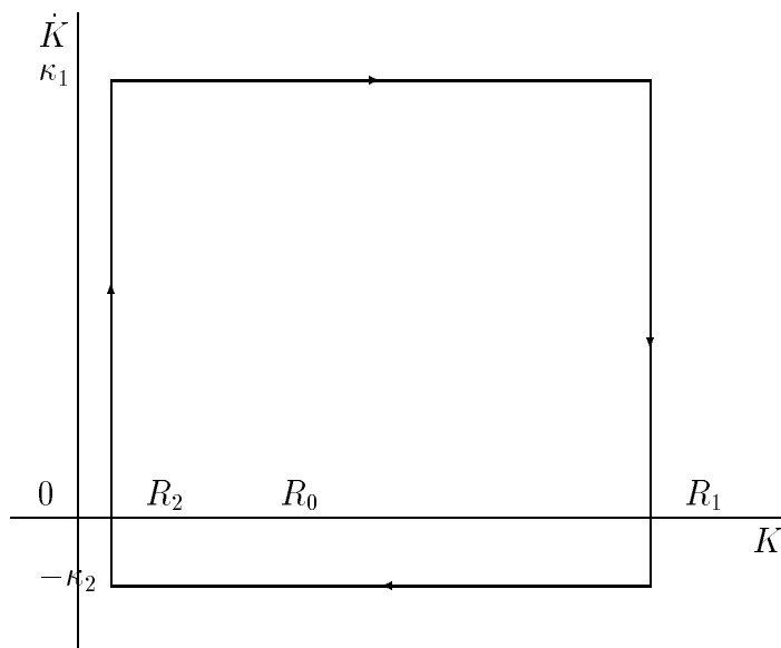
図 8.3: グッドウィンのモデルの位相図 1
