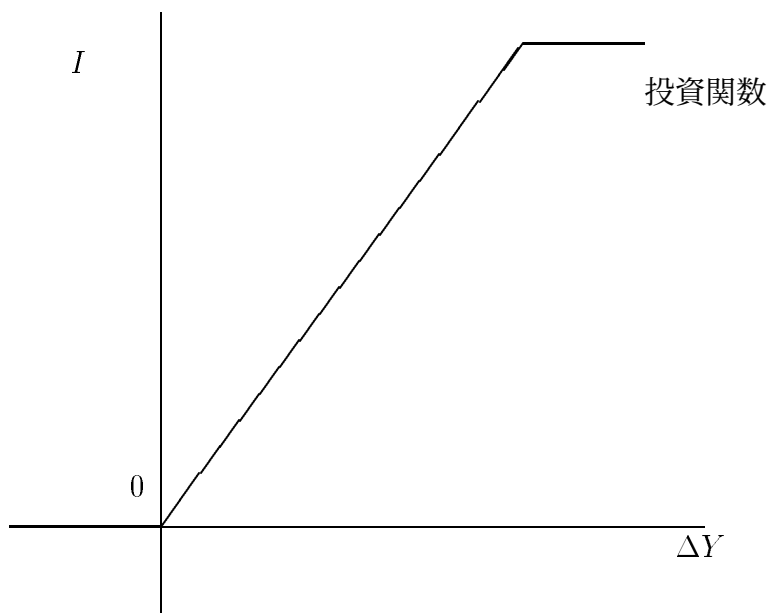
図 8.1: ヒックスの床-天井モデルの投資関数
